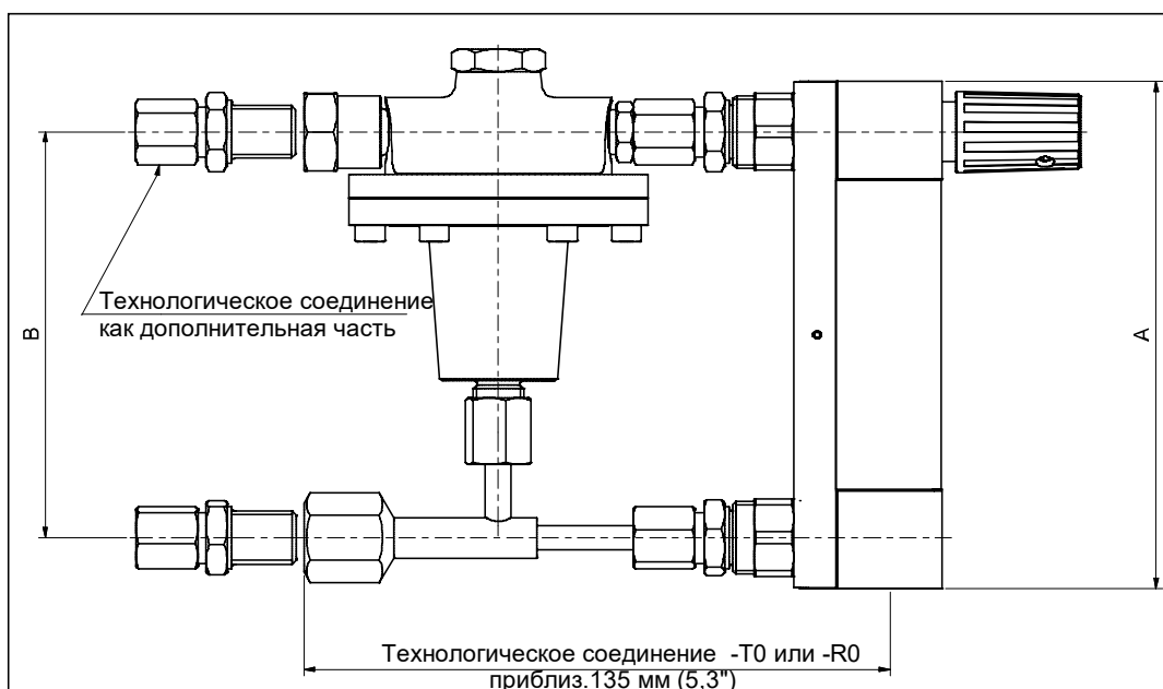
Рис. 8. Версия с выпускным клапаном и опцией контроллера выходного расхода /R3
